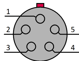
Abb. 13: CANSAS Buchse (Basiseinheit) (Sicht auf die Buchse)
