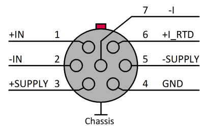
Abb. 15: UTI-6 Buchse (Belegung) (Sicht auf die Buchse)
