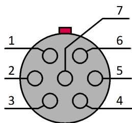
Abb. 12: GPS Buchse (Basiseinheit) (Sicht auf die Buchse)
