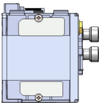
linke Modul-Seite mit Haltevorrichtung für die Abdeckungen der Modul Steckverbinder
